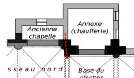
Figure 94 – Renforcement du piédroit Nord au droit de l'arc fracturé
