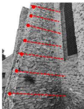
Figure 93 – Condition d'harpage des deux contreforts Sud à assurer (voir préconisations)
